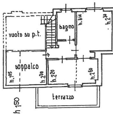
PIANO PRIMO (SOTTOTETTO)
